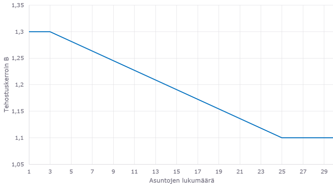
Kuva 10.1. Asuntokohtaisella ilmanvaihdon tehostuksella varustetun asuinrakennuksen keskitetyn ilmanvaihdon tehostuskerroin
