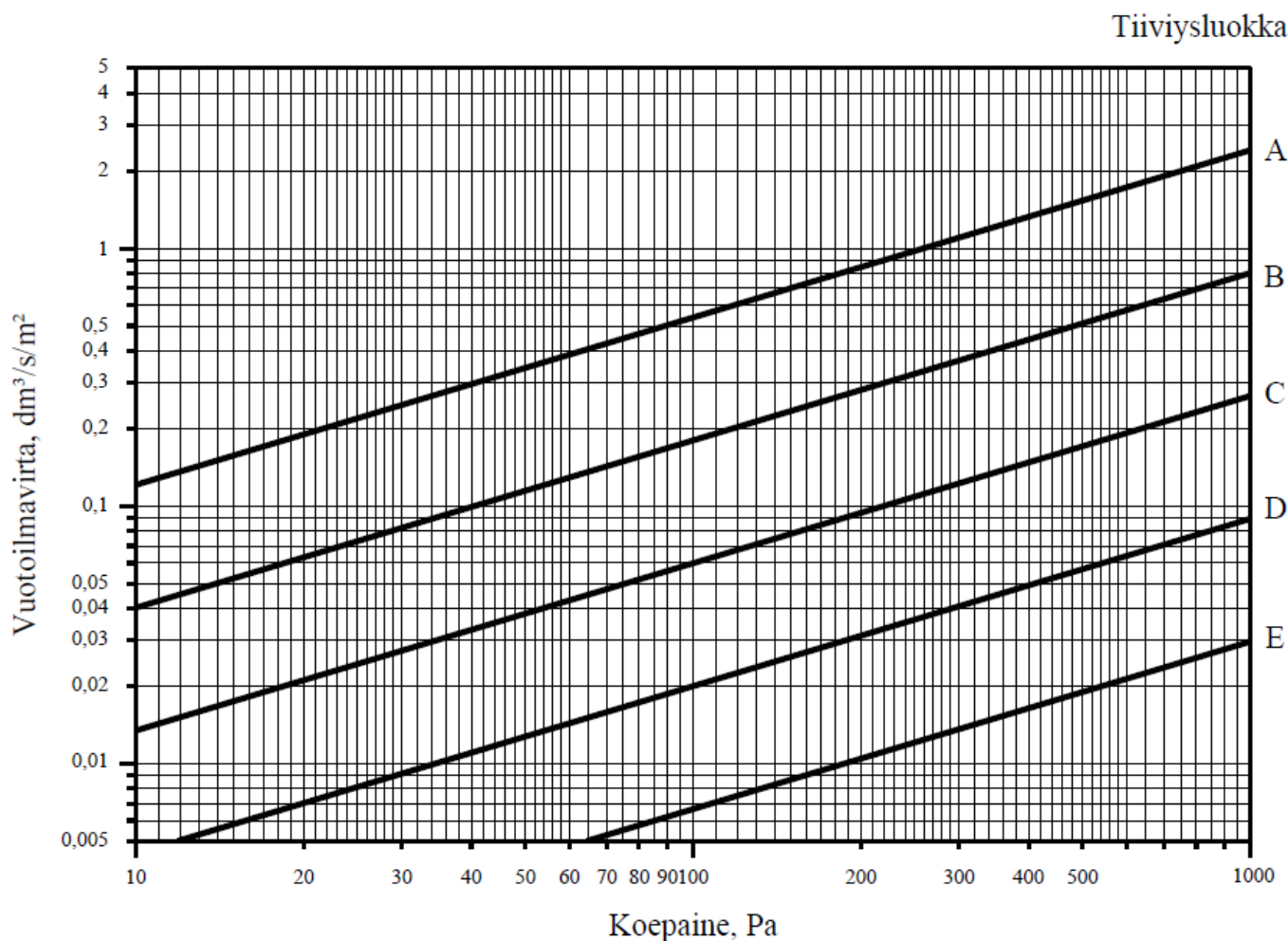
Kuva 19.1 Ilmanvaihtojärjestelmän ja sen osien suurimmat sallitut vuotoilmavirrat vaipan pinta-alaa kohti
