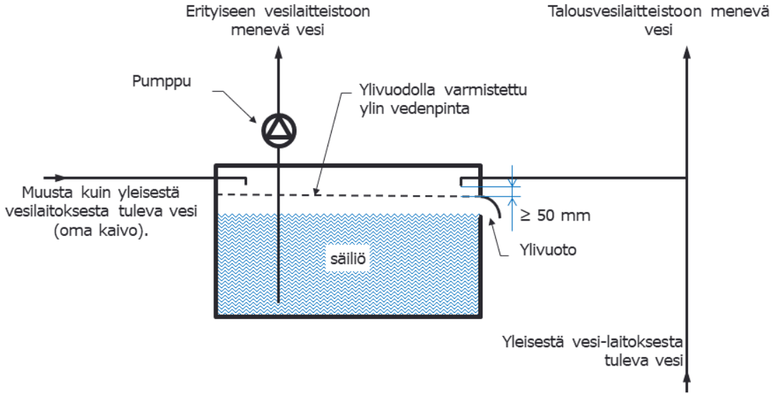
Kuva 5.1. Esimerkki veden johtamisesta vesihuoltolaitoksen verkosta ja muusta vesilähteestä käyttäen takaisinimusuojauksella AB.
