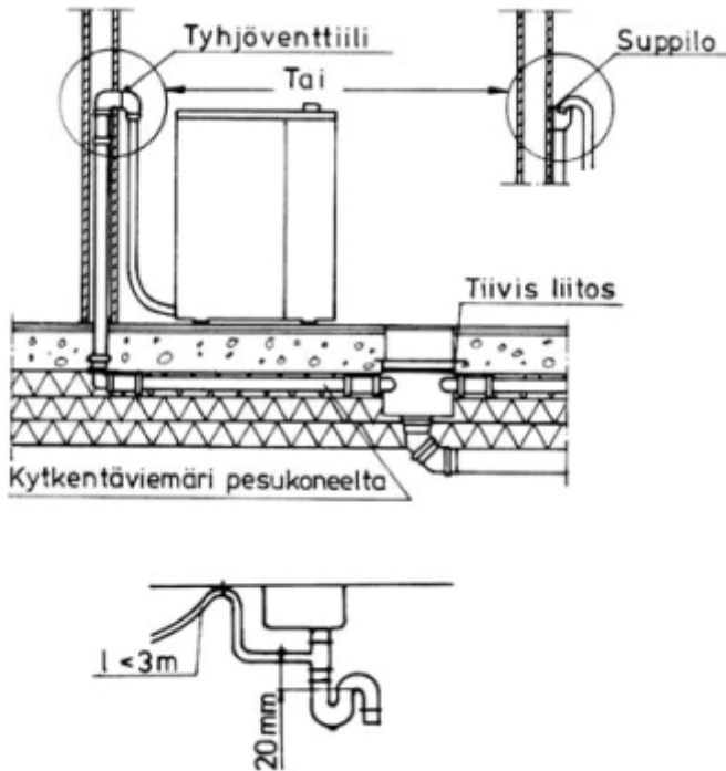
Kuva 29.1 Esimerkkejä kotitalouskäyttöön tarkoitetun pesu- tai astianpesukoneen viemäröintitavoista.
