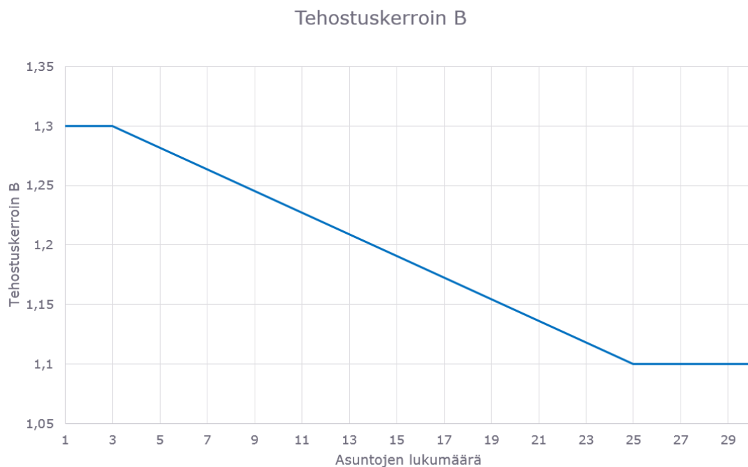
Kuva 10.1. Asuntokohtaisella ilmanvaihdon tehostuksella varustetun asuinrakennuksen keskitetyn ilmanvaihdon tehostuskerroin
